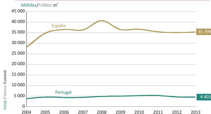
81 Importação de gás natural, 2004-2013 Natural gas imports, 2004-2013
